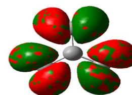
HOMO
