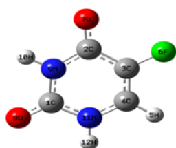
Fig. 1. 5-Fluorouracil
