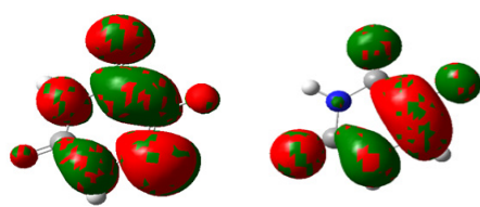
LUMO
