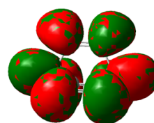
LUMO
